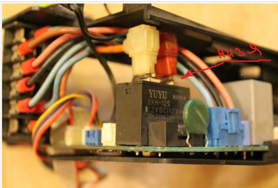
Закорочные контакты пускового реле. Практический ремонт платы управления | Неисправное реле кондиционера (сплит-системы) от Замыкания силовых контактов, плата управления.
